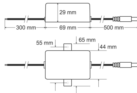
Rys. 1 Widok mechaniczny zasilacza.
